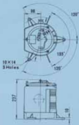
引船燈 型式 A2-ST Towing Light
