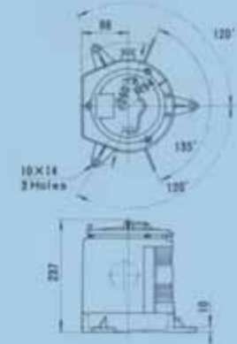
船尾燈 型式 A2-SS Sternlight
