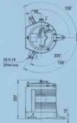
しやう燈 型式 A2-SM Masthead Light
