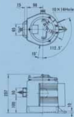
げん燈 型式 A2-SLR Sidelight
