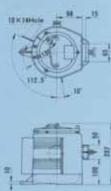
げん燈 型式 A2-SRG Sidelight
