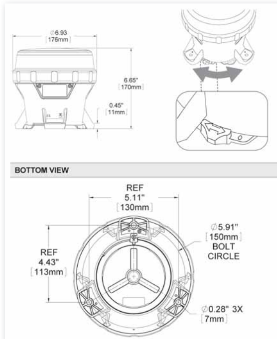
Caramanah M650 4NM
