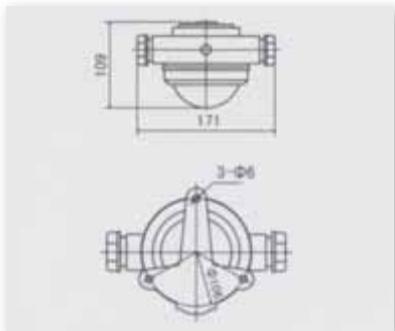
Candescent pendant light
